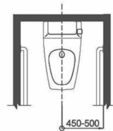
การเข้าถึงโกส้วมชนิดนั่งราบ สำหรับผู้พิการที่ไม่ได้ใช้เก้าอี้ล้อเลื่อน
