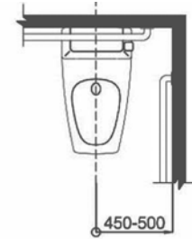
การเข้าถึงโกส้วมชนิดนั่งราบ สำหรับผู้พิการที่ใช้เก้าอี้ล้อเลื่อน
